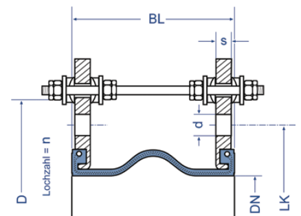
innere und äußere Kugelenkverspannung
