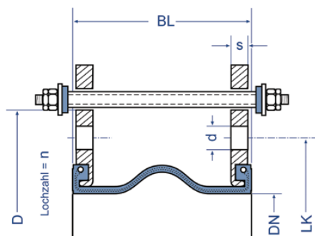
Zugbegrenzung
