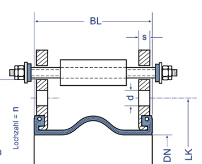
Zug- / Schubbegrenzung
