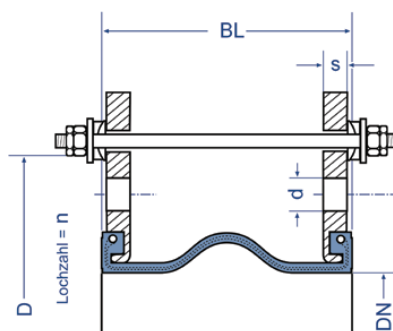
äußere Kugelenkverspannung
