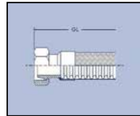
Dichtkegel mit Ü-Mutter
