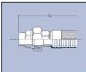
Dreiteilige Verschraubung konischdichtend Außengewinde
