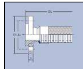
V-Bund mit Losflansch
