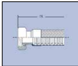
Milchrohr Verschraubung Kegelstutzen mit Nutmutter DIN 11851
