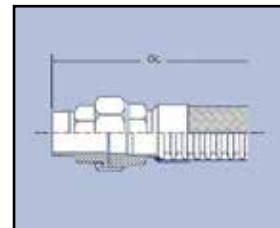
3-teilige Verschraubung flachdichtend Außengewinde
