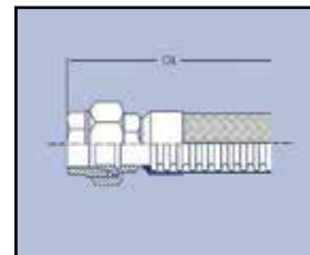
Dreiteilige Verschraubung konischdichtend Innengewinde
