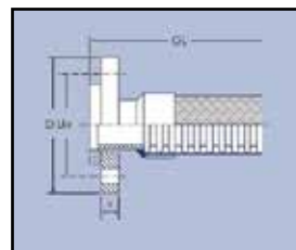
Glatter Bund mit Losflansch
