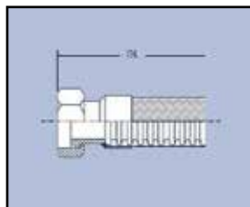
Flachdichtender Stutzen mit Ü-Mutter
