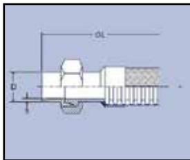
3-tlg. 24° Verschraubung mit AE
